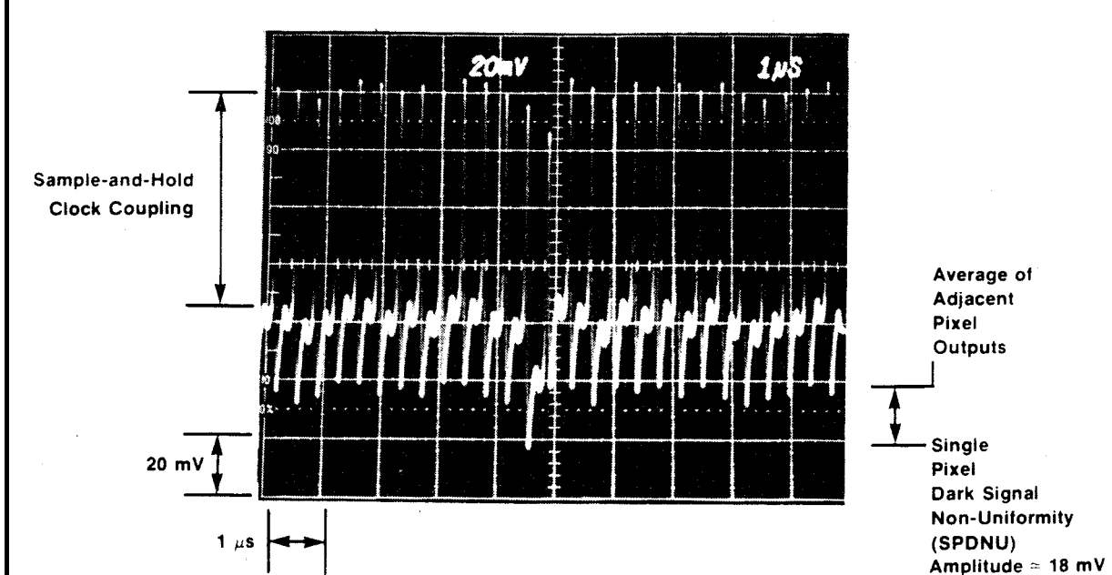
Fig. 6 DARK SIGNAL PARAMETERS (DS)
